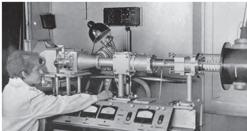
И.Е. Грибова у электронографа (слева). С.В.Каверин у блока питания электронографа
